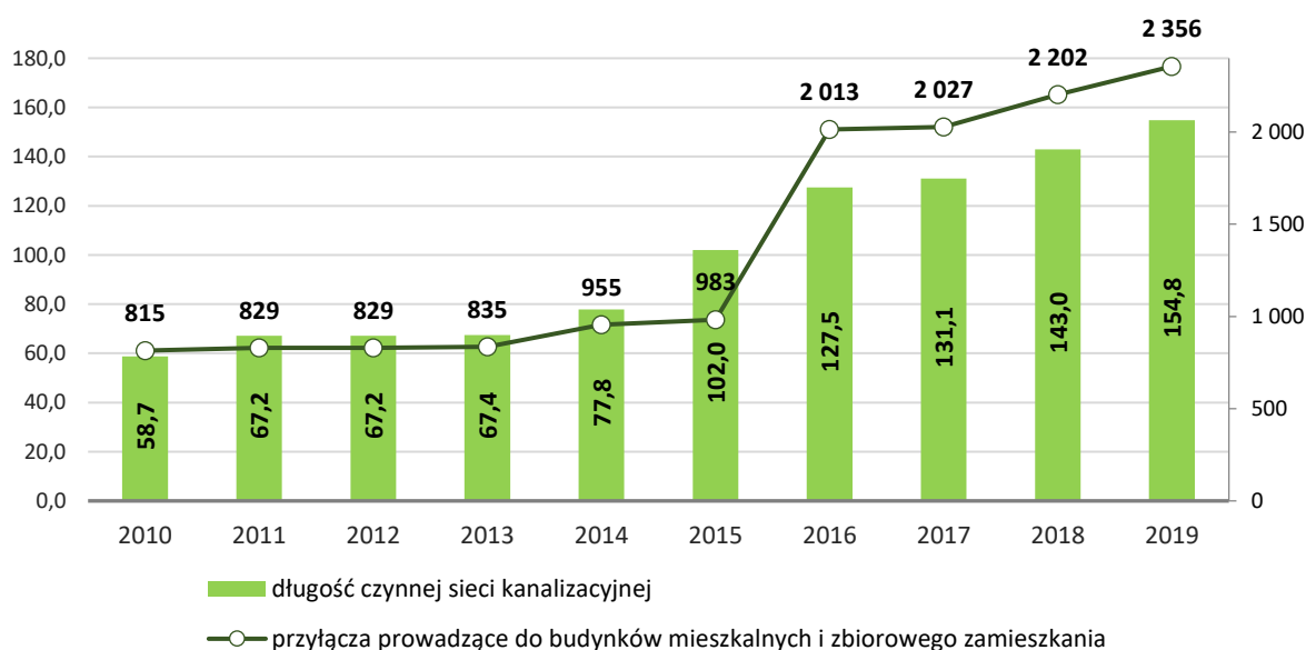
Wykres 19. Długość rozdzielczej sieci wodociągowej oraz liczba przyłączy prowadzących do budynków na terenie Gminy Biłgoraj w latach 2010-2019 (km, szt.)
