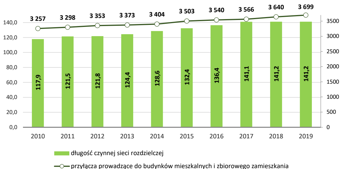
Wykres 17. Długość rozdzielczej sieci wodociągowej oraz liczba przyłączy prowadzących do budynków na terenie Gminy Biłgoraj w latach 2010-2019 (km, szt.)
